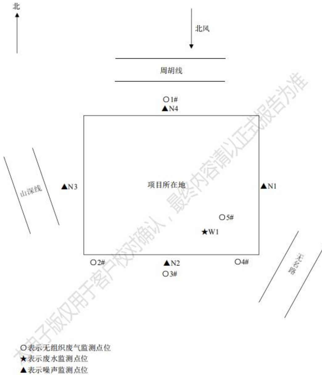
图 3.2-1 验收监测采样点位示意图
